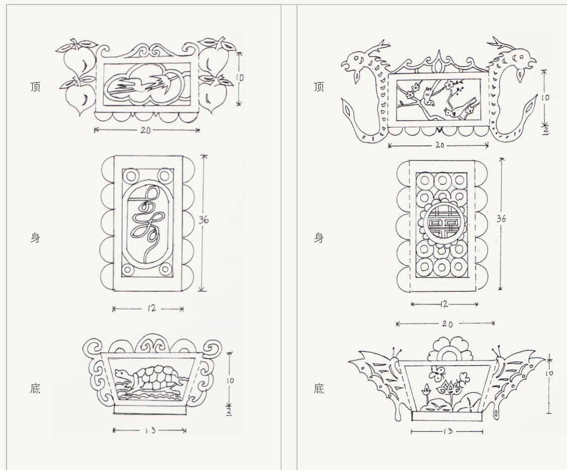
“寿”灯灯面设计图（单位：cm）
