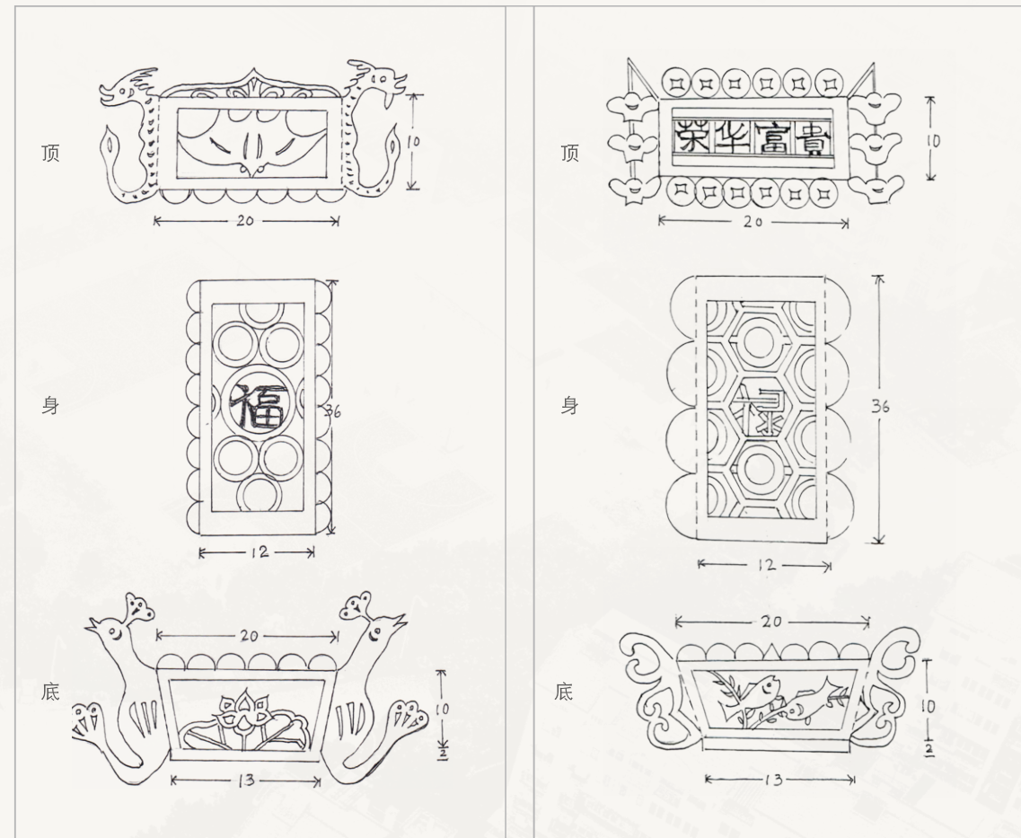
“福” 灯灯面设计图 (单位: cm)
