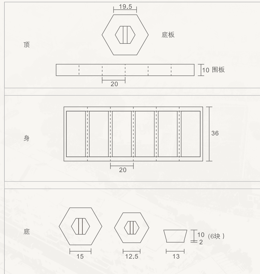
“福” “禄” “寿” “喜” 骨架设计图 (单位: cm)
