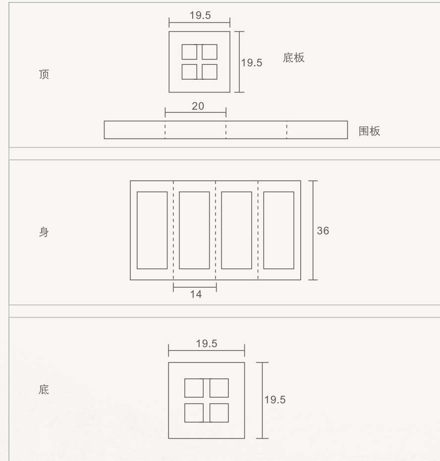
十二生肖骨架设计图（单位：cm）
