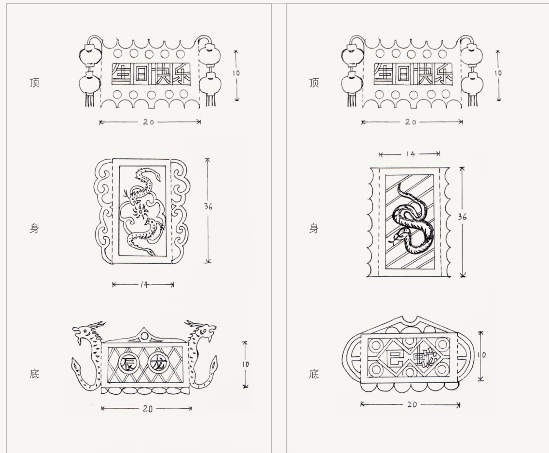
十二生肖（龙）灯面设计（单位：cm）
