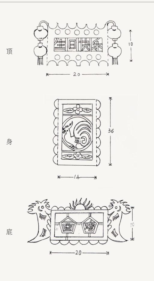
十二生肖（鸡）灯面设计（单位：cm）
