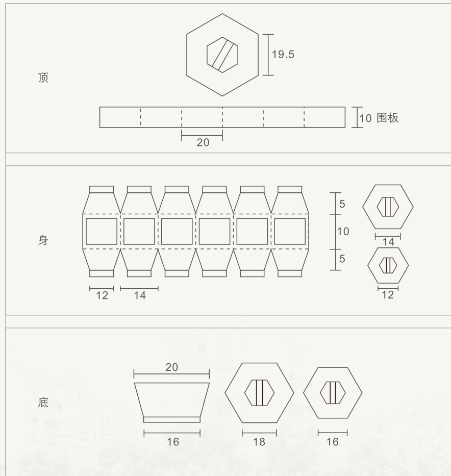
“社会主义核心价值观”灯骨架设计 (单位: cm)
