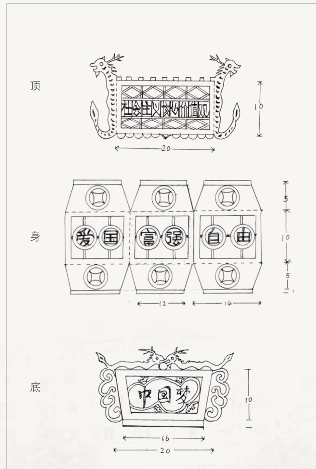
“社会主义核心价值观”灯面设计 (单位: cm)
