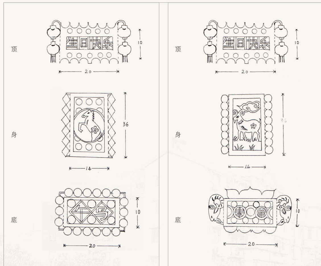
十二生肖 (马) 灯面设计 (单位: cm)
