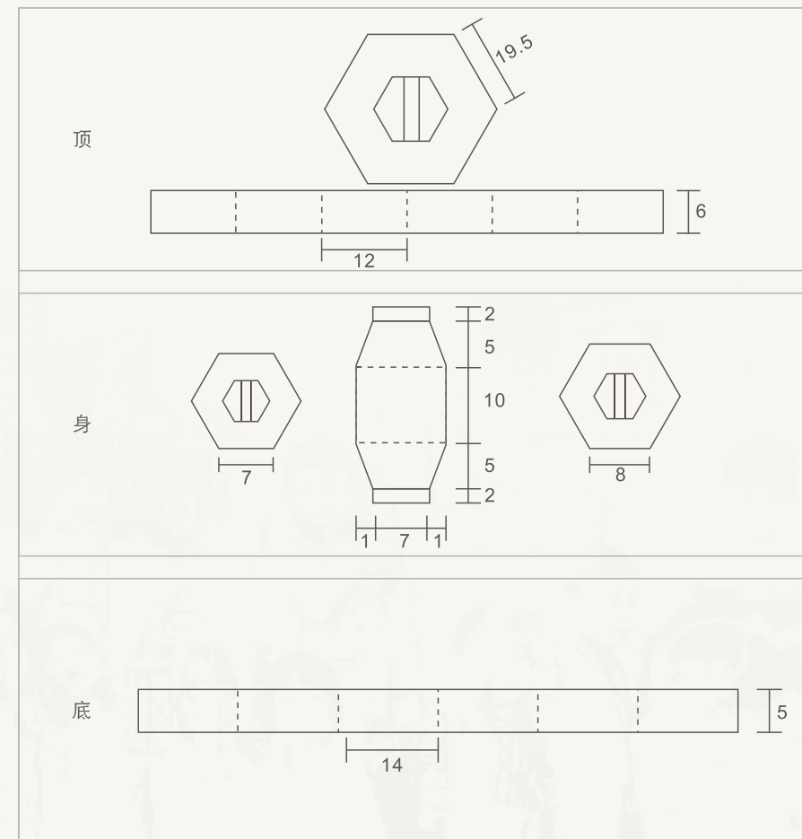
“万事如意” 宫灯骨架设计图（单位：cm）
