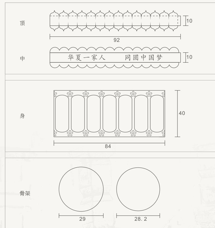
“华夏一家人”宫灯设计图（单位：cm）
