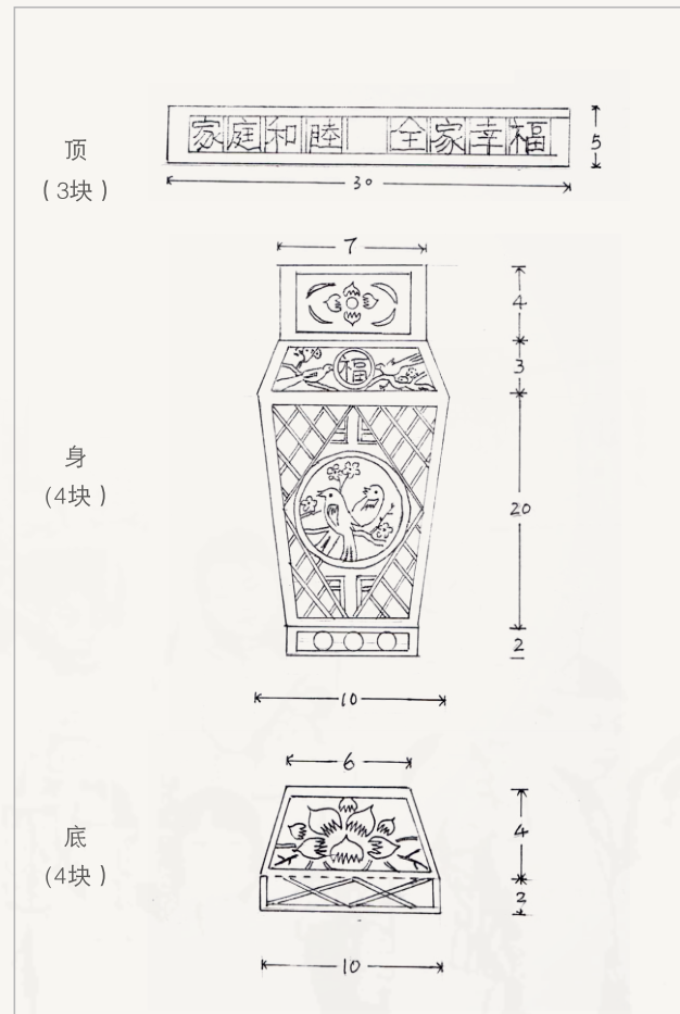
“家和万事兴” 宫灯灯面设计（单位：cm）
