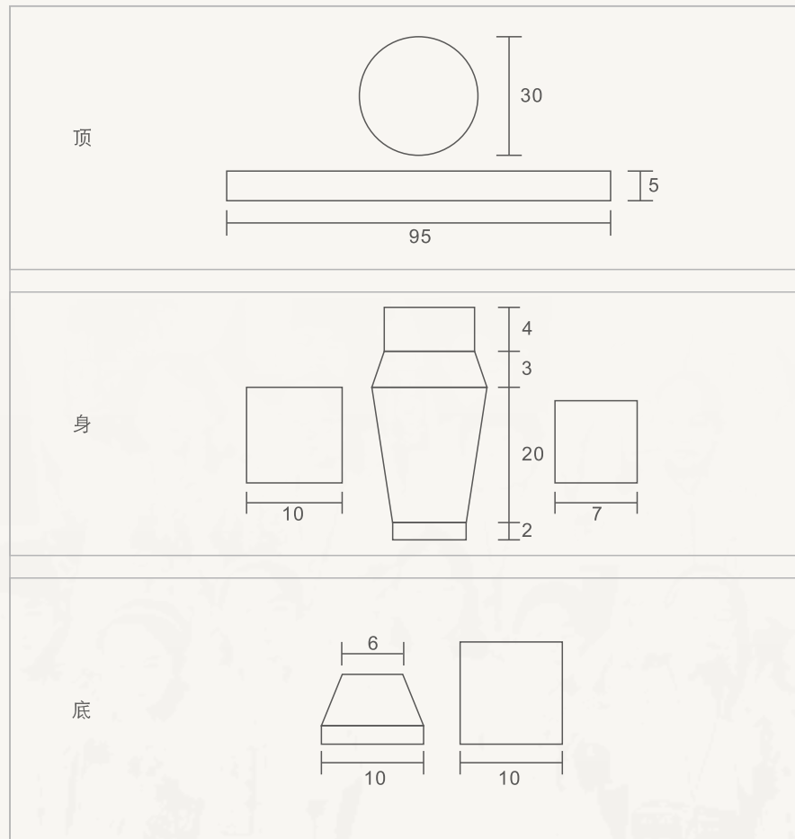
“家和万事兴” 宫灯骨架设计图（单位：cm）
